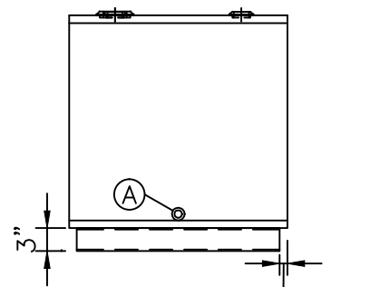
LEFT SIDE
