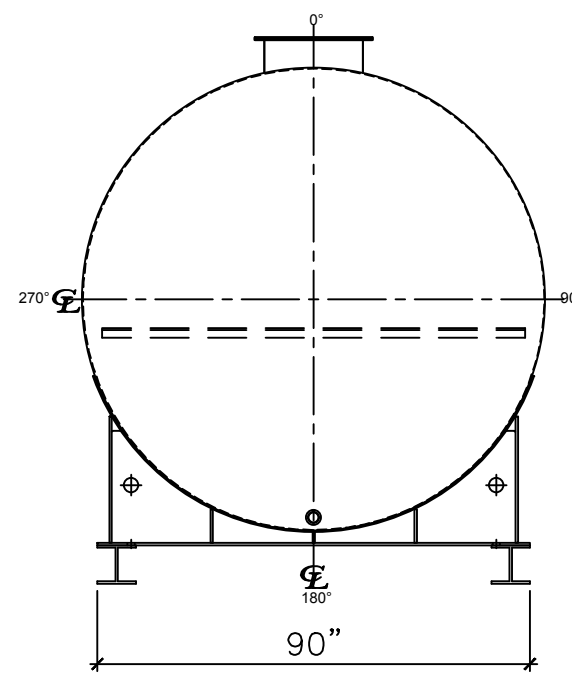
LEFT SIDE
