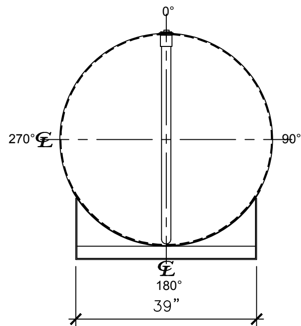
LEFT SIDE
