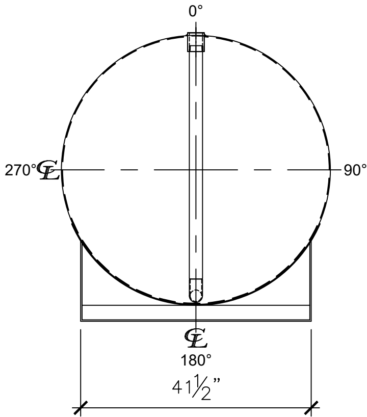
LEFT SIDE
