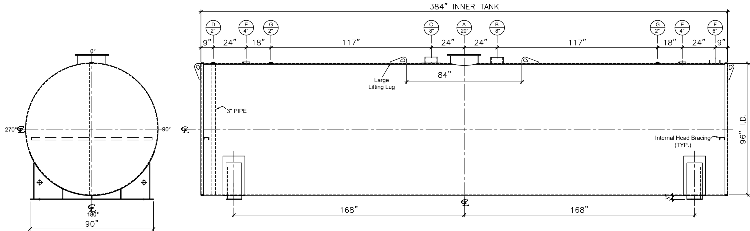
LEFT SIDE
